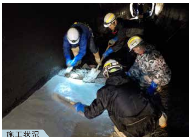
導水路トンネル インバート補修
